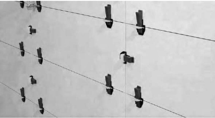
Ejemplo de colocación del Sistema de Nivelación Rls en Revestimiento(fig.10) y Pavimento (fig.11)
